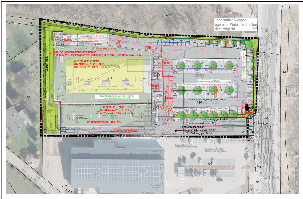
Abbildung 17: Planung zum geplanten Lebensmittelvollsortimenter mit integriertem Backshop und Café sowie Drogeriemarkt o.M. und genordet
